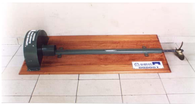
FIGURA 8 - Protótipo do dispositivo de segurança
